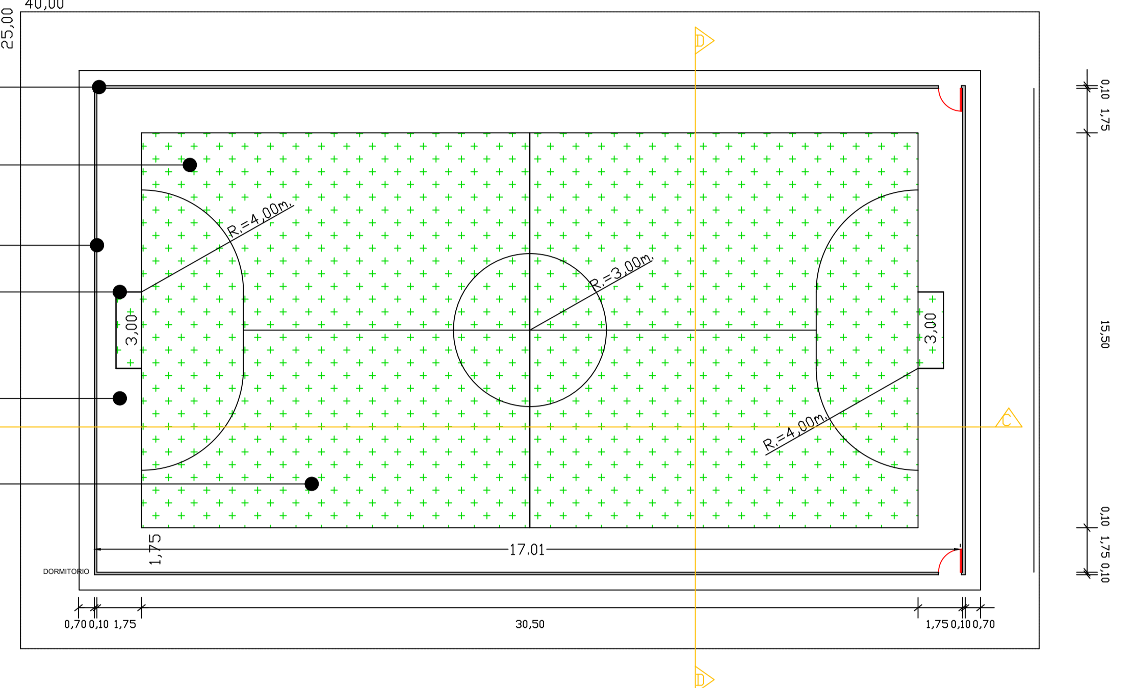
PLANTA BAIXA - DEMARCAÇÃO DE ESPORTE
